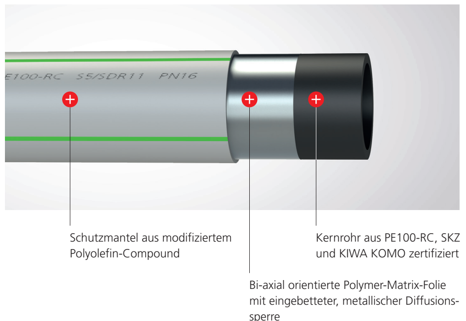
2 Aufbau des Rohres
